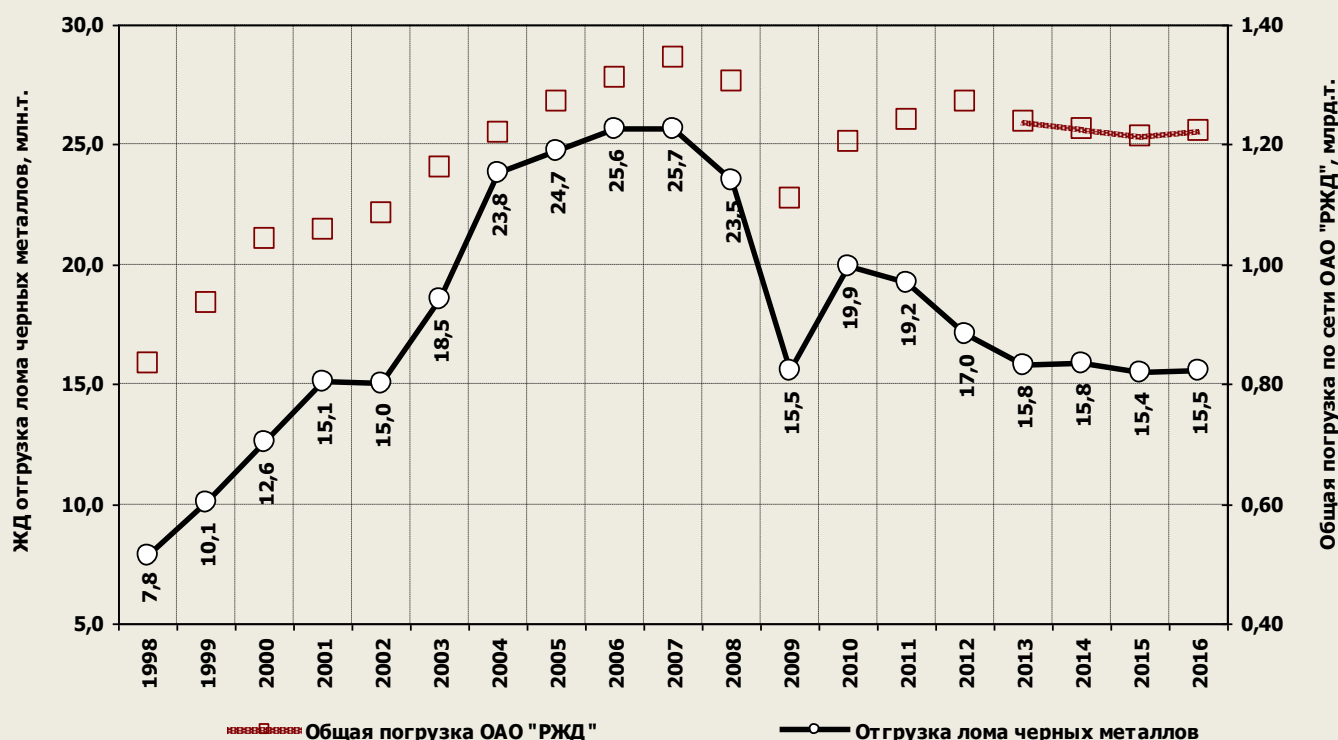
Рисунок 3 - Сравнение динамики общей погрузки по сети ОАО «РЖД» и отгрузки металлолома
