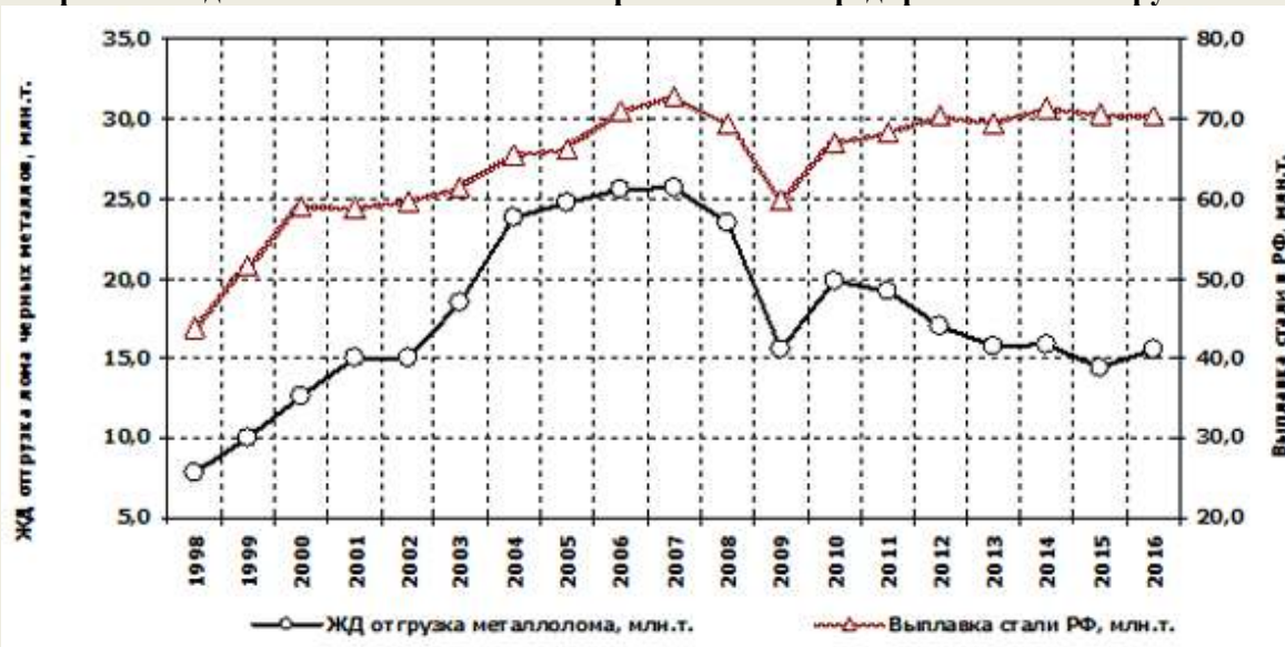
Рисунок 2- Структура и динамика отгрузок лома черных металлов железнодорожным транспортом за период 1998-2016 гг.
